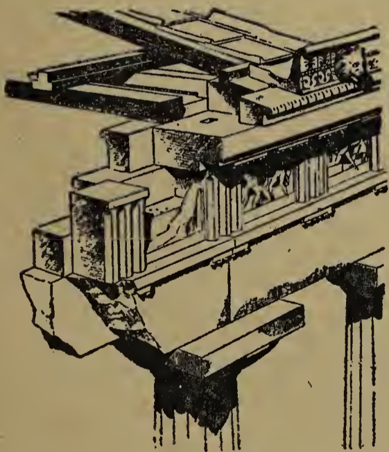
FIGURA 262—(Reconstrucción de Viollet-le-Duc). Capiteles y entablamento del Partenón.
